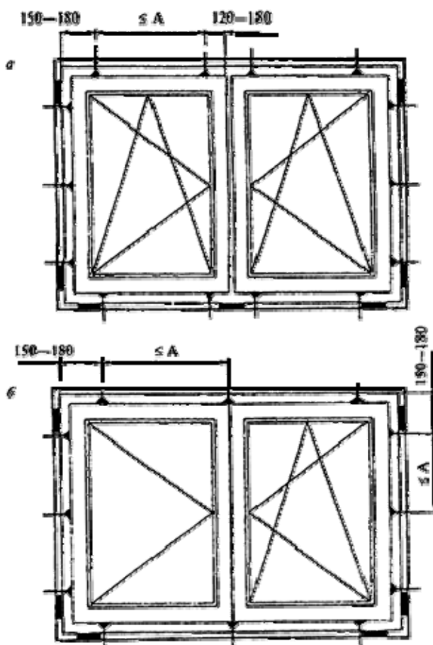
а - оконный блок с вертикальным импостом; б - оконный блок с безимпостным (штильповым) притвором; А - расстояние между крепежными деталями
